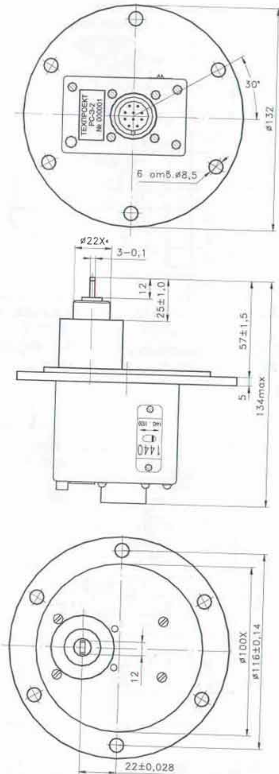
Рисунок 1 - Присоединительные размеры РС-Э
