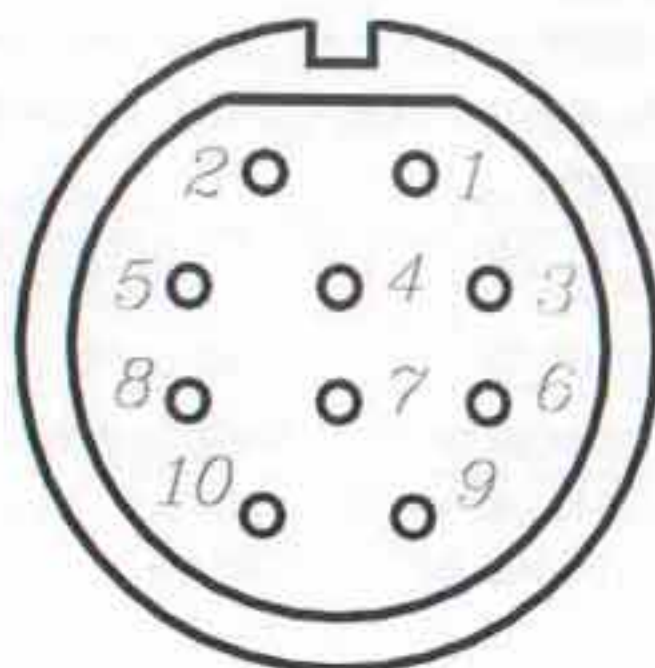
Рисунок 7 - Нумерация контактов соединителя со стороны пайки
